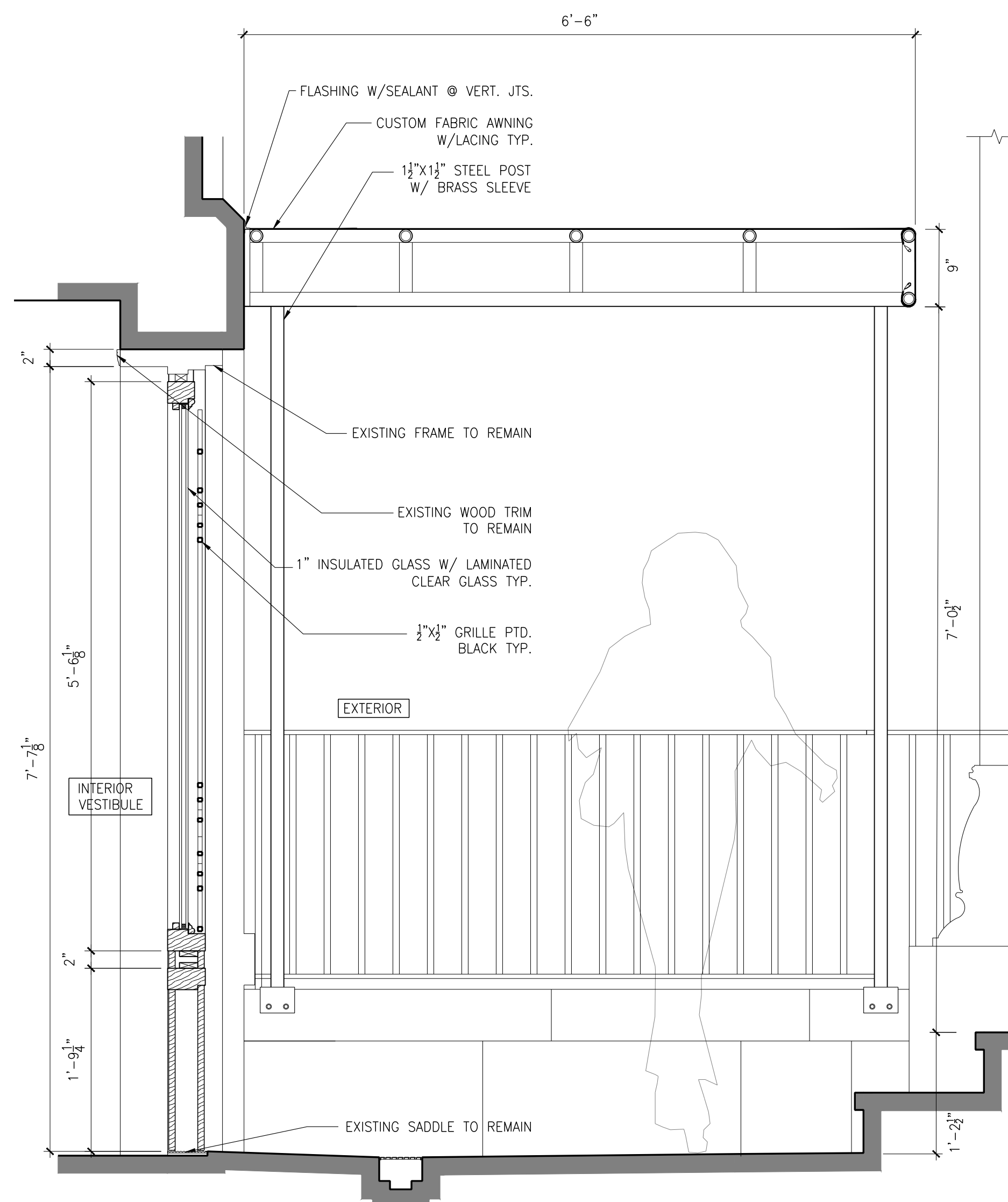
1 SIDELITE DETAIL SCALE: 1" = 1'-0"
