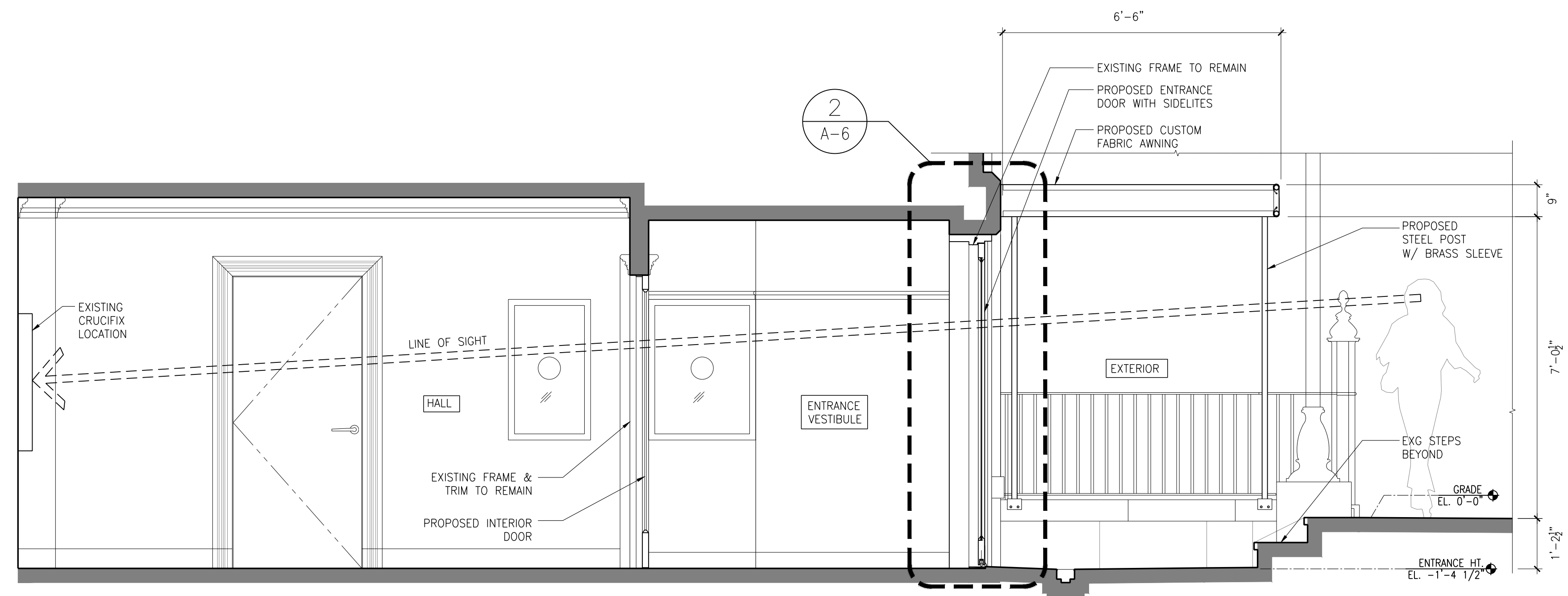
2 CROSS SECTION SCALE: 1/2" = 1'-0"
